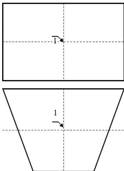
Рисунок 7.13 - Точка удара для закаленных плоских стекол
