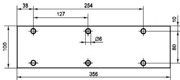
Рисунок 7.22 - Испытуемый образец
