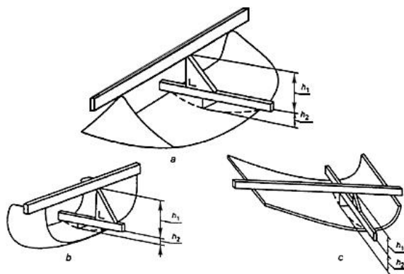
Рисунок А.1 - Определение высоты сегмента
