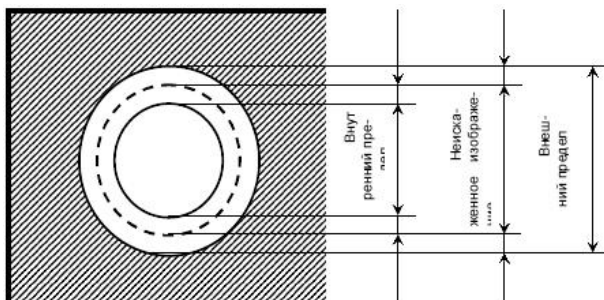
Рисунок 7.5 - Контрольный шаблон
