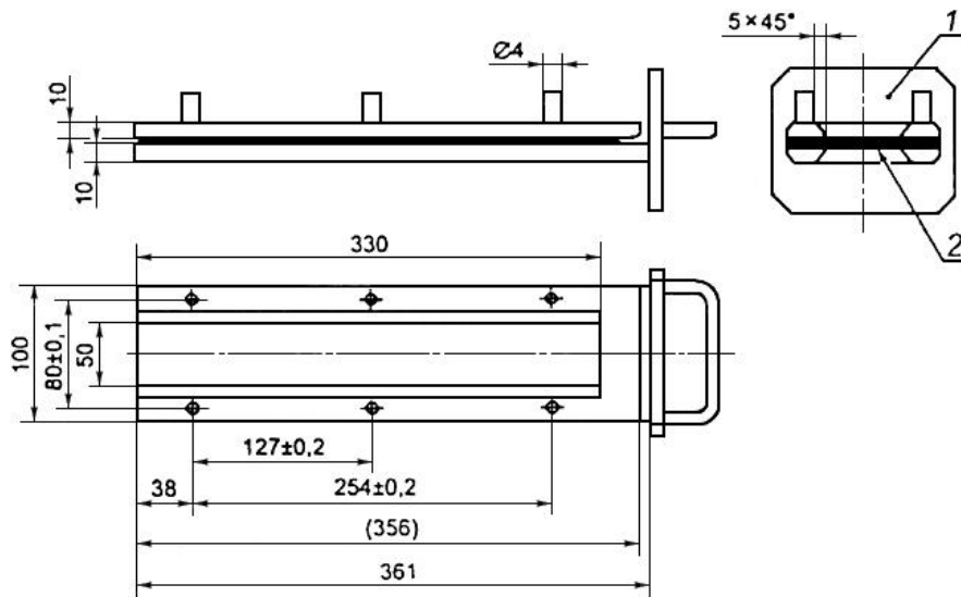
Рисунок 7.20 - Схема подставки
