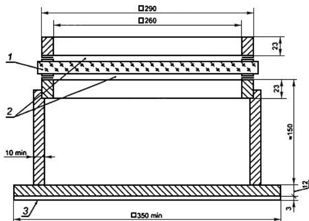
Рисунок 7.10 - Подставка для испытания с помощью шара
