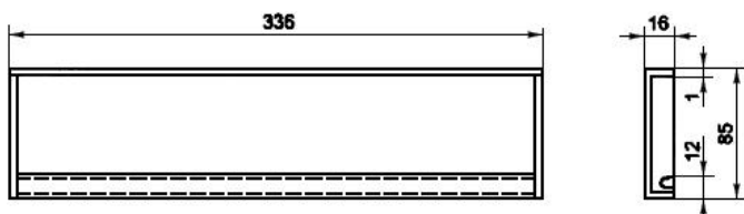
Рисунок 7.19 - Ванночка
